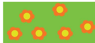
Slika 11: translacijska simetrija
