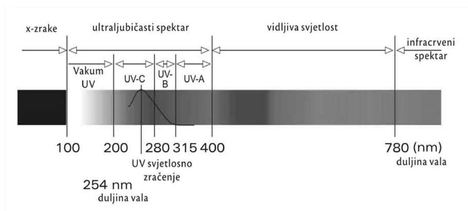
Slika 4.1: Svjetlosni spektar [3]
