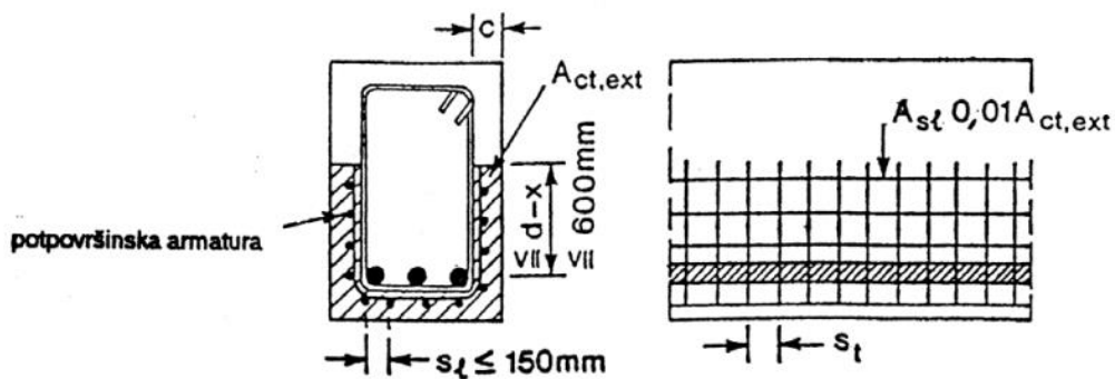
Slika 4.7: Potpovršinska armatura
