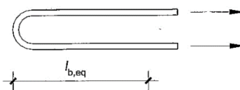
d) Jednakovrijedna duljina sidrenja za standardnu petlju
