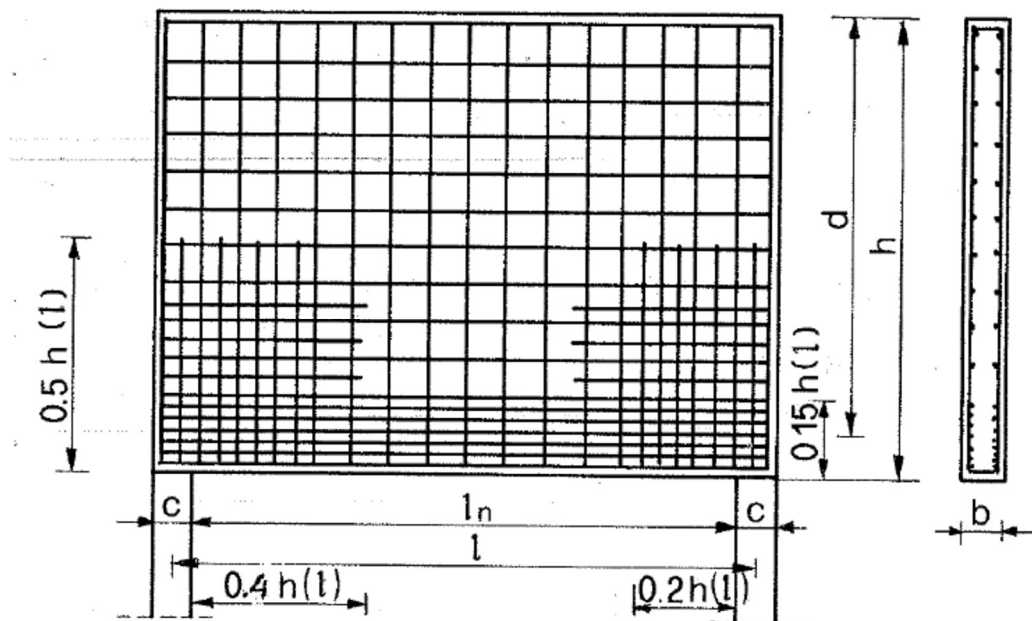
Slika 2.3.1. Armiranje zidnog nosača
