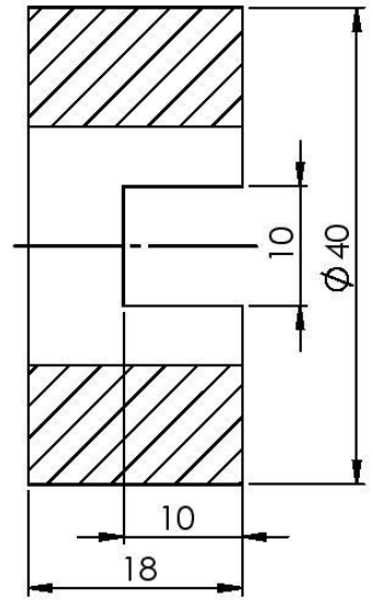
PRESJEK A-A
