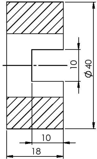
PRESJEK A-A
