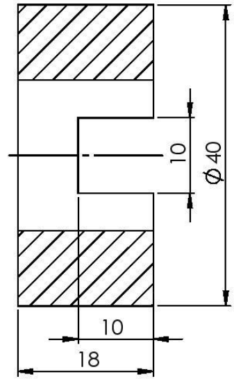
PRESJEK A-A
