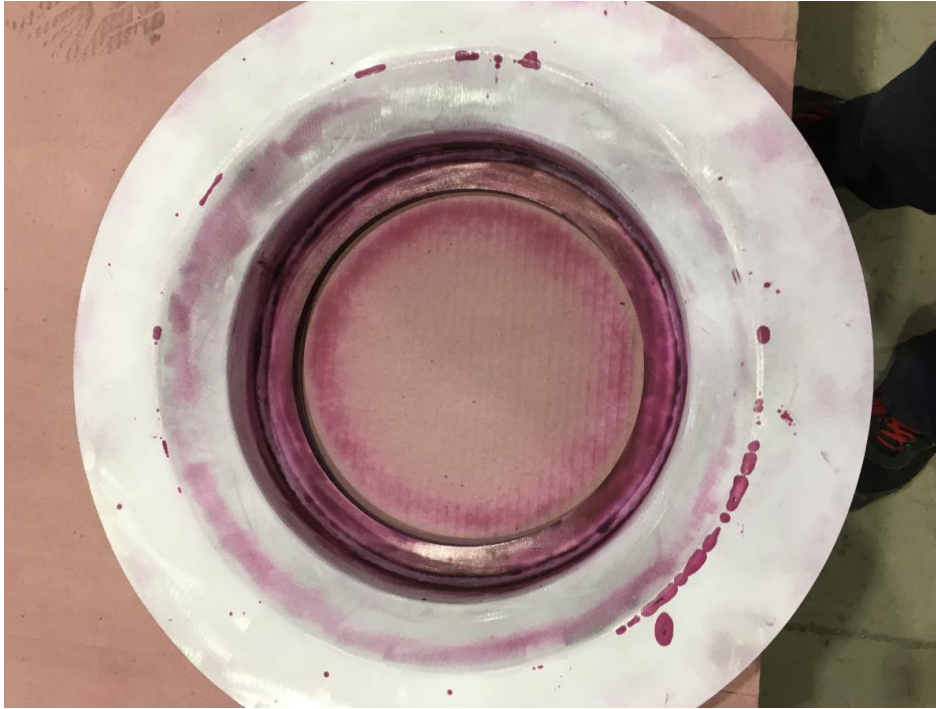
Slika 34: Ispitivanje zavarenog spoja penetrantima (faza prikaza indikacija)
