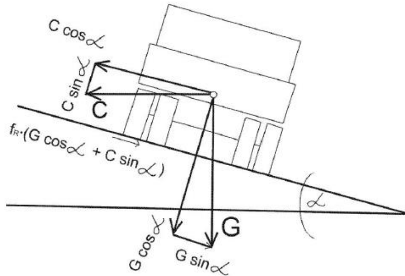
Slika 6. Stabilnost vozila u krivini (Rezo, 2016.)
