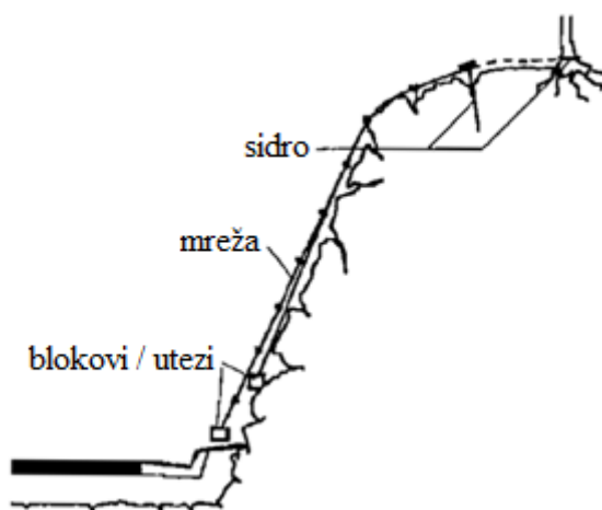
Slika 2.6. Žičana mreža
