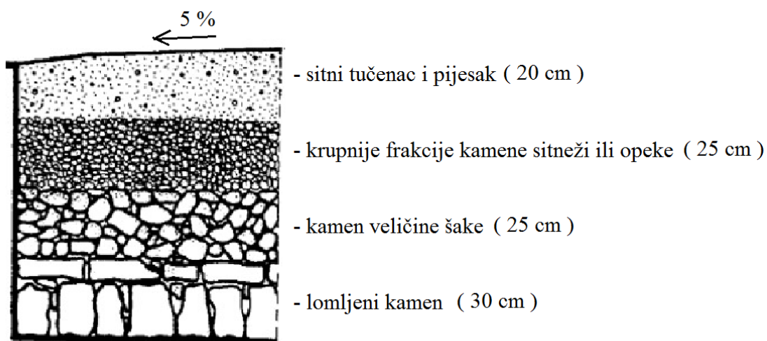
Slika 1: Poprečni presjek rimske ceste
