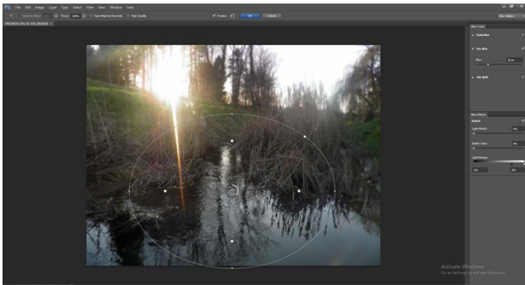
Slika 9.1 'Iris Blur'
