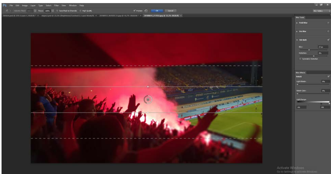
Slika 9.2 Blur; 'Tilt-Shift'
