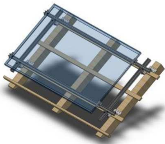
Slika 4.14. Jednostruki nosač (lijevo) i dvostruki nosač (desno)
