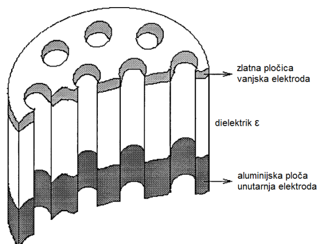
Slika 2.10. Senzor vlage[10]
