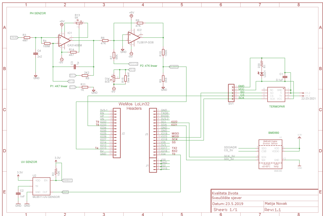
Slika 3.1. Shema spoja
