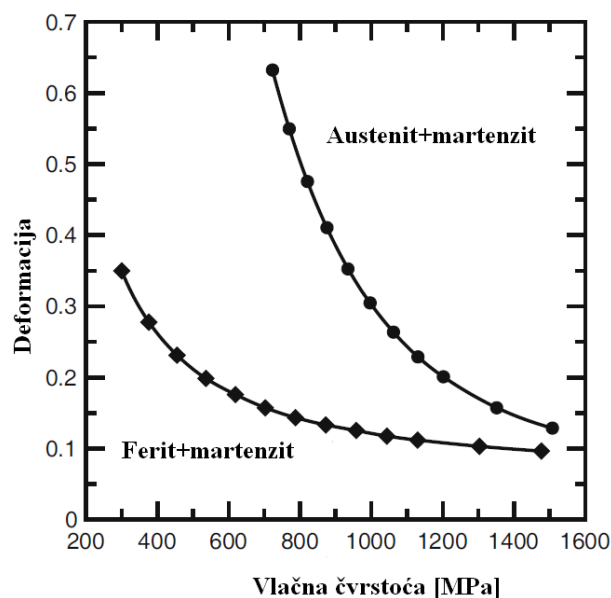
Dijagram 3.20 Odnos vlačne čvrstoće i deformacije za različite mikrostrukure [25]
