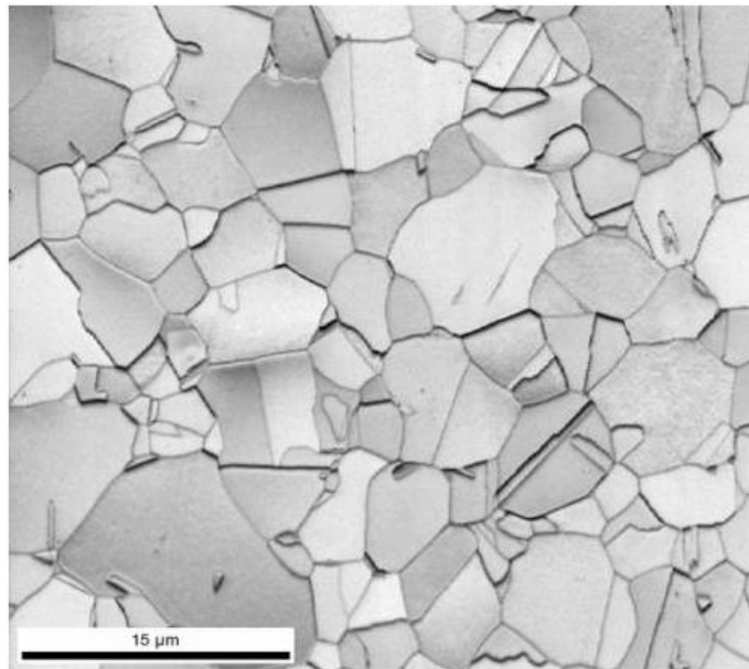
Slika 3.16 Mikrostruktura TWIP čelika [39]
