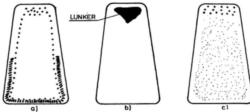
Slika 1.4 Presjek ingota: a) nesmiřeni, b) smireni, c) polusmiřeni [10]
