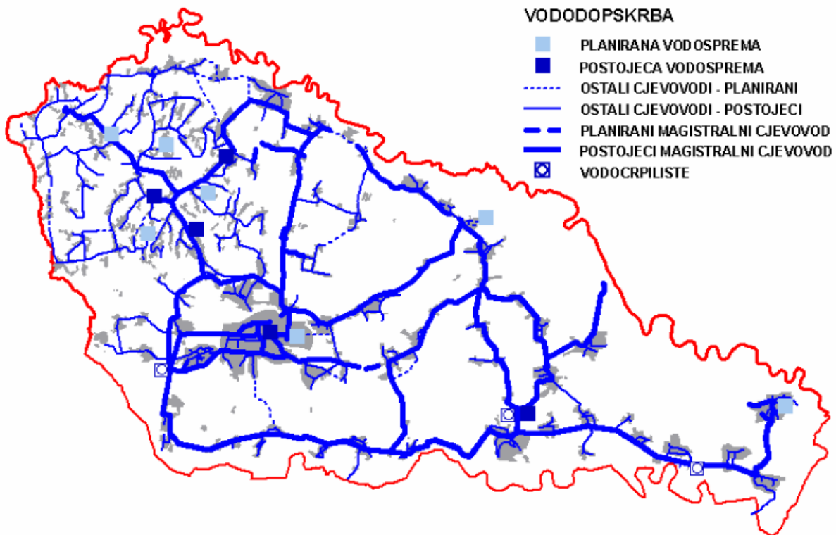
Slika 1.1 Shematski prikaz vodoopskrbnog sustava Međimurske županije [1]
