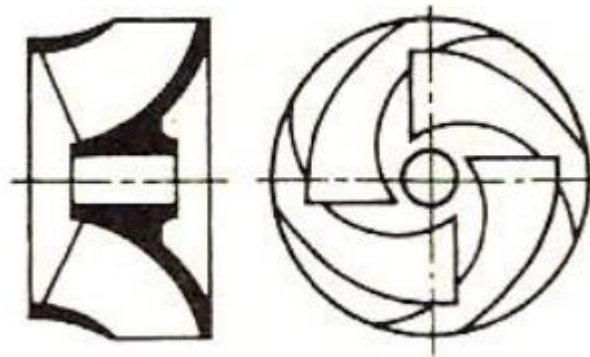
Slika 3.6 Dijagonalno radno kolo[7]
