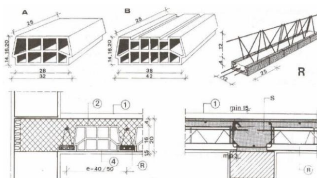
Slika 2.17 Izometrija ispune i gredice i presjek fert stropa
