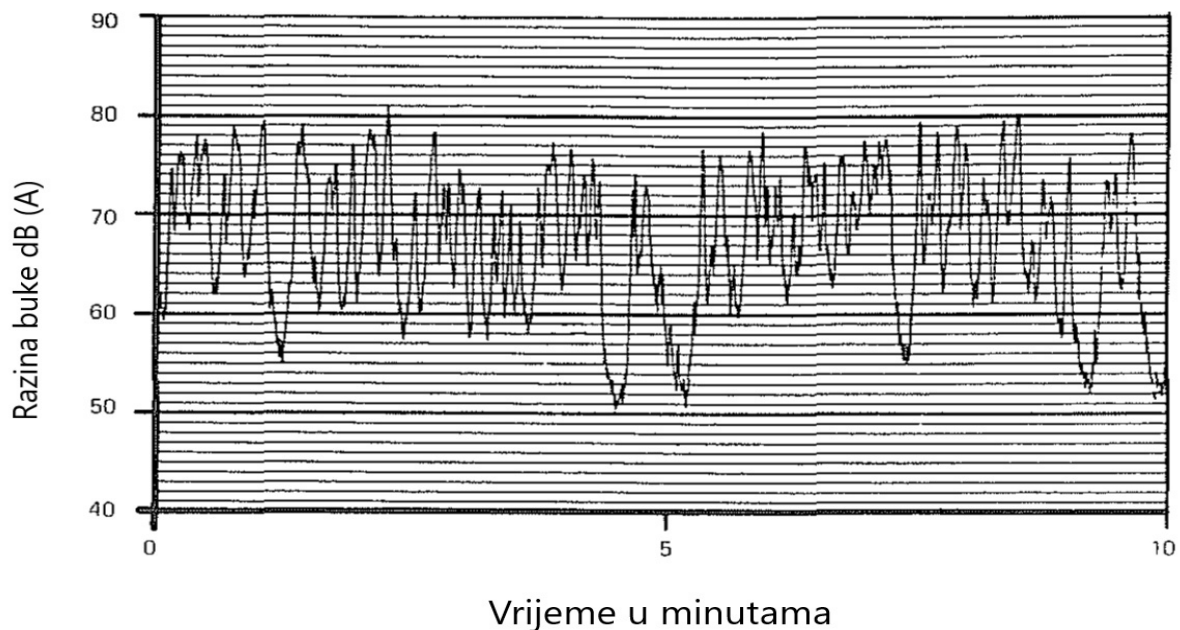
Slika 1. Razina buke kod podloge od betonskog kolnika (Izvor: Gottfried Nievelt, Gerhard Stehno, Helmut Stickler, Johann Ertl- Noise level reduction through silent asphalt )
