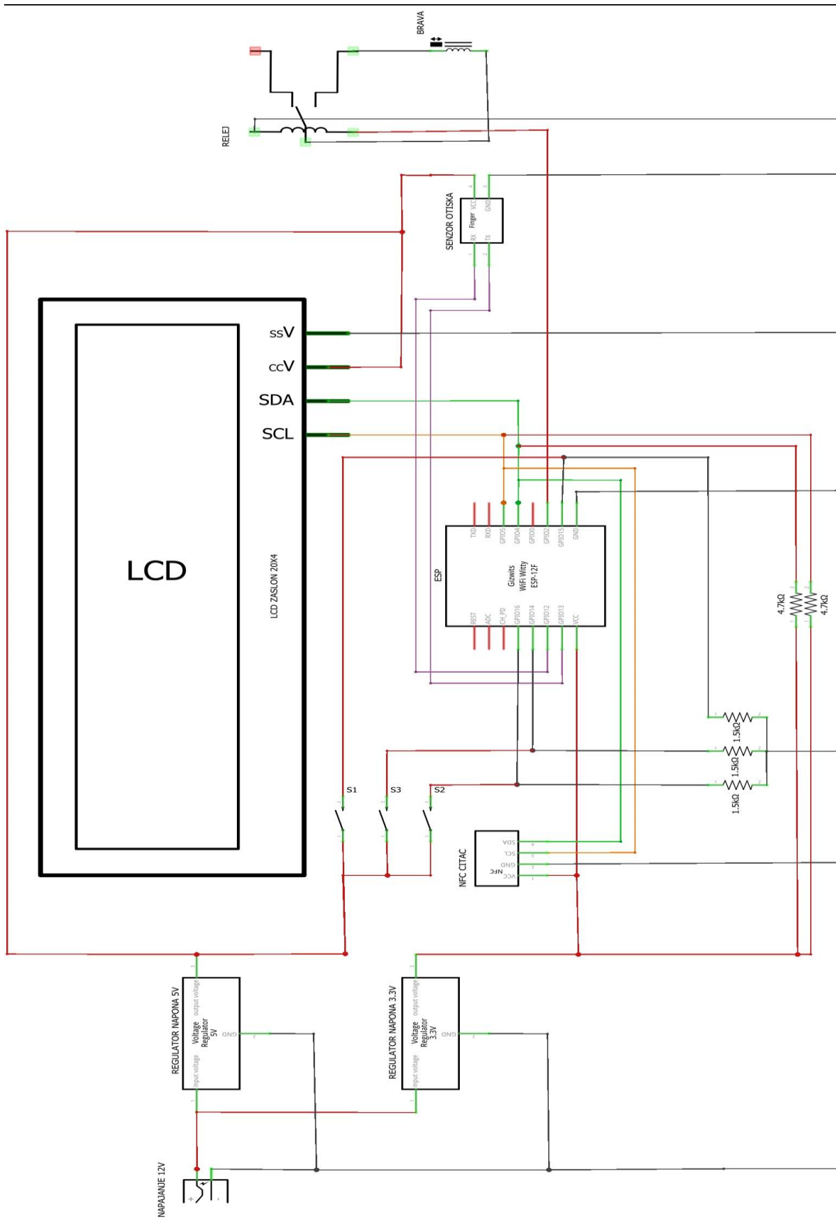
Slika 9: Shema sklopa
