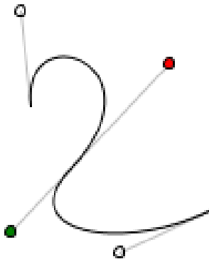
Slika 5.3.6.7: Glatko kontinuirane krivulje A i B
