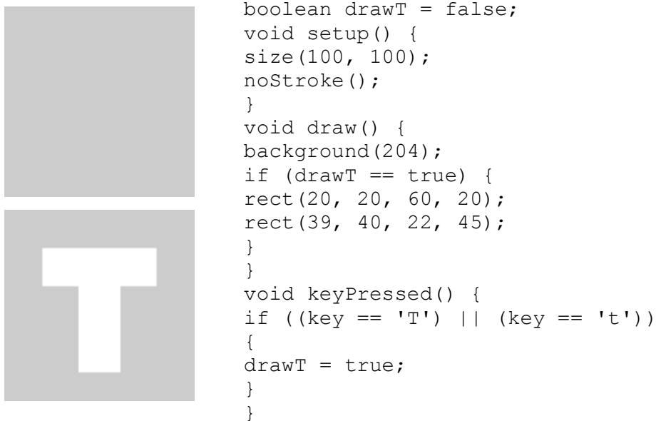
Slika 5.3.3.23: Mijenjanje vrijednosti varijable drawT
