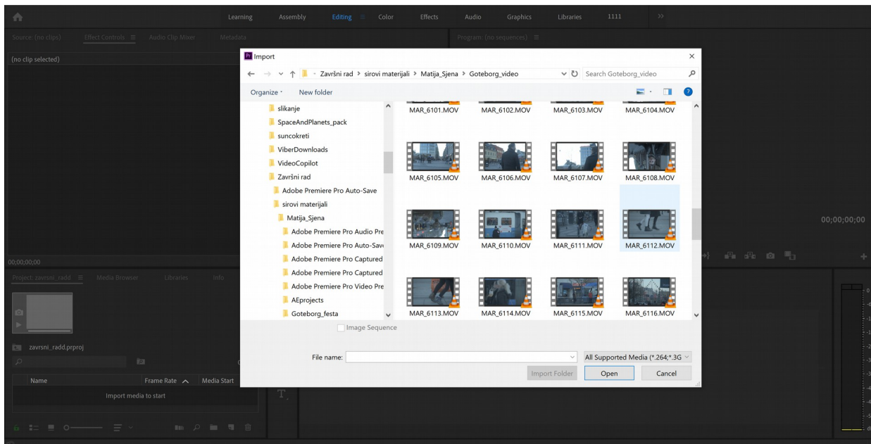
Slika 8.2. - Uvoz datoteka
