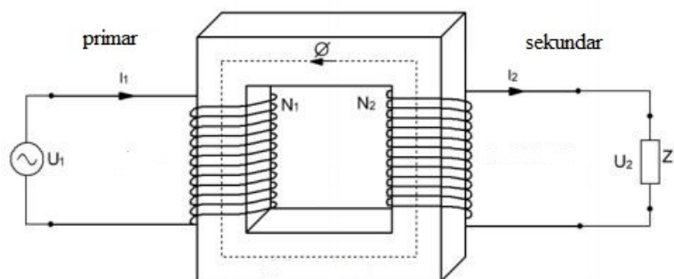
Slika 3.7 Shema transformatora
