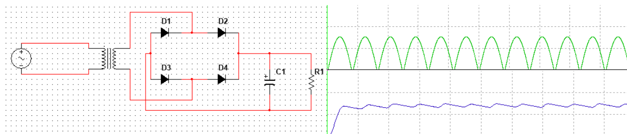
Slika 4.6 Shema spoja Greatzovog spoja s kondenzatorom za filtriranje napona i izgled filtriranog napona
