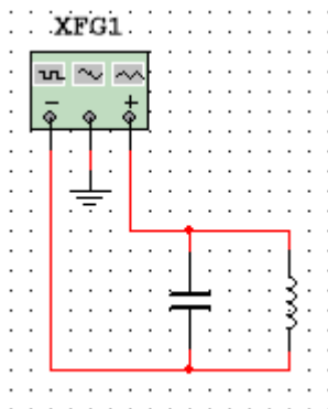
Slika 5.3 Shema spoja primarnog kruga
