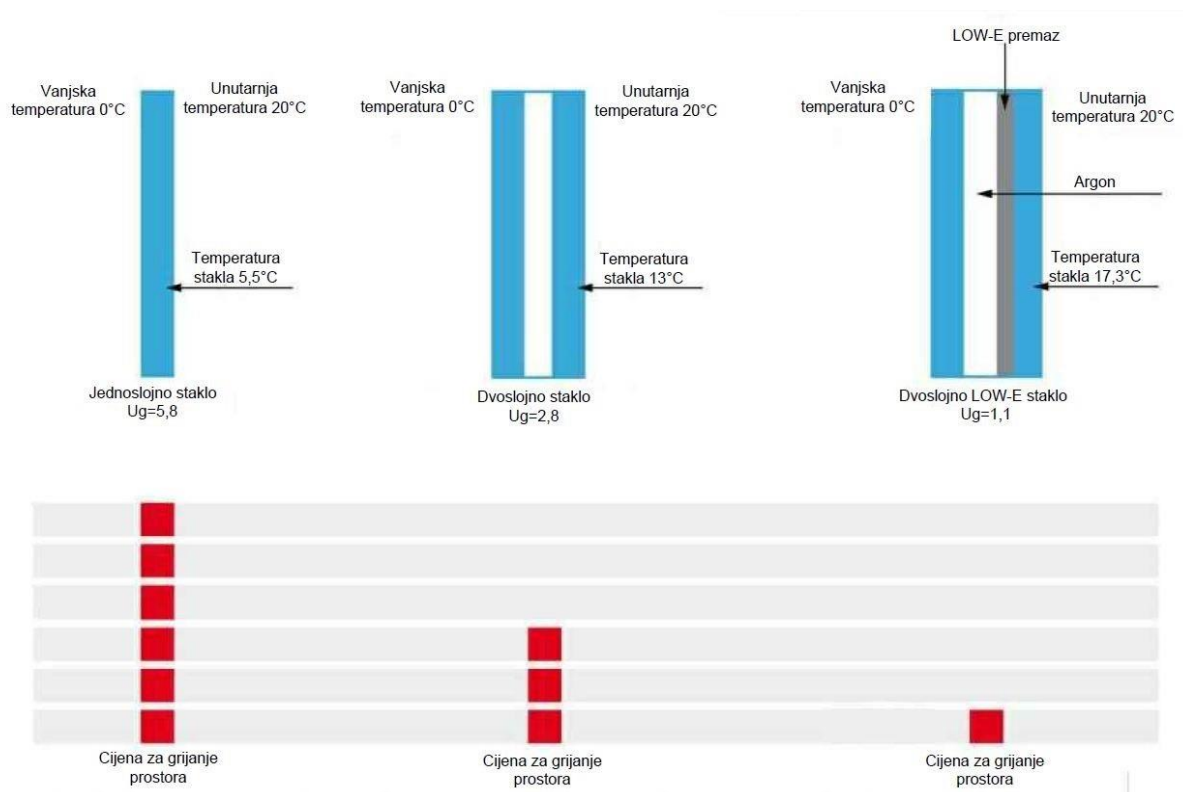
Slika 3.17. Usporedba jednoslojnog i dvoslojnog stakla
