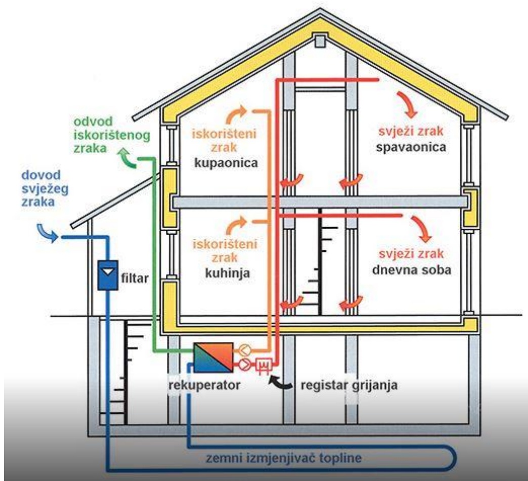
Slika 3.22. Ventilacija niskoenergetske kuće
