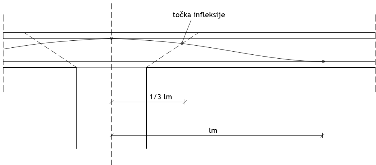
Slika 2.14. Shematski prikaz slobodnog vođenja kabela
