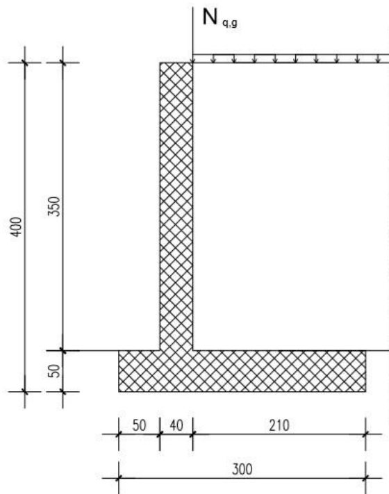
Slika 14.: AB-zid
