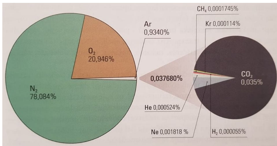
Slika 5. Sastav zraka
