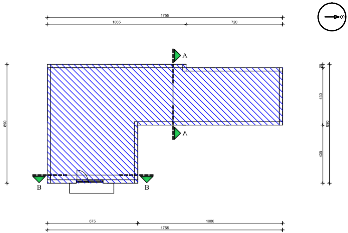
Slika 5.1.3.2 Tlocrt tavana
