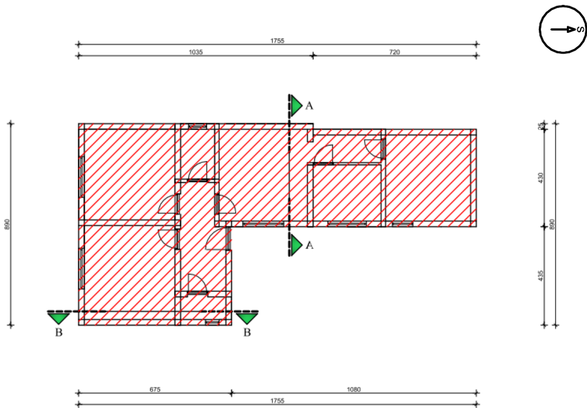
Slika 5.1.3.1 Tlocrt prizemlja
