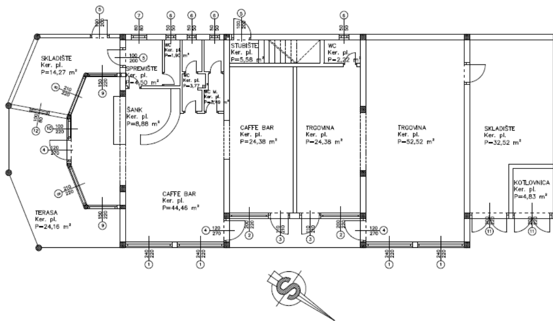
Slika 3 Tlocrt prizemlja
