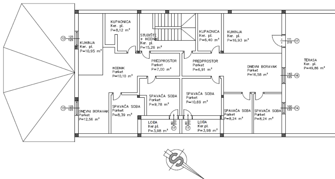
Slika 4 Tlocrt kata
