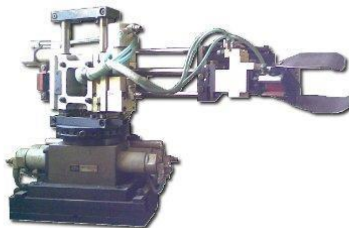
Slika 2-10 Cilindrični robot [21]
