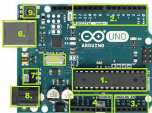
Slika 2-1. Arduino Uno R3 model i najbitniji dijelovi
