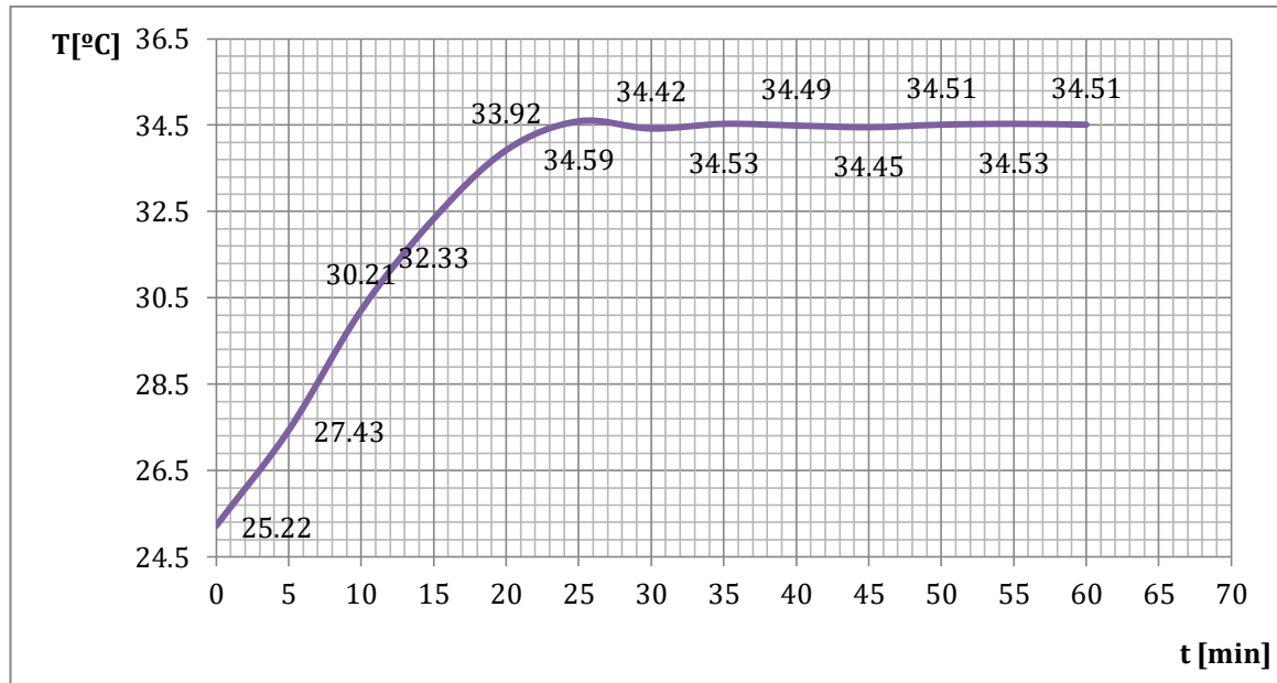
Slika 5.5. Graf Mjerenje temperature komore u dnevnom boravku (25 °C) s jednom žaruljom
