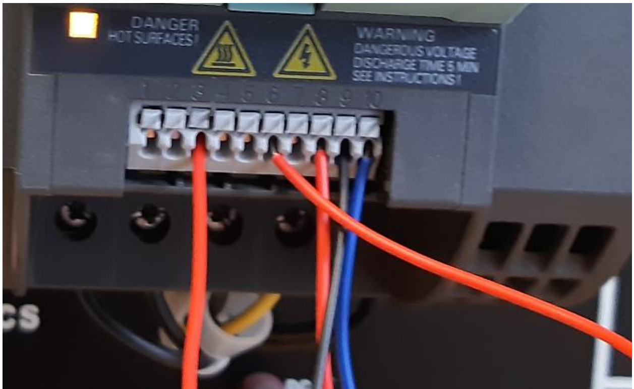
Slika 5.1 Shema terminala[7]
