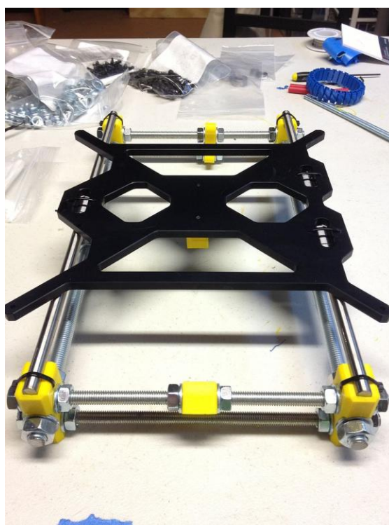
Slika 32. Y os Pruse i3 MK3- tiskani dijelovi prikazani su žutom bojom
