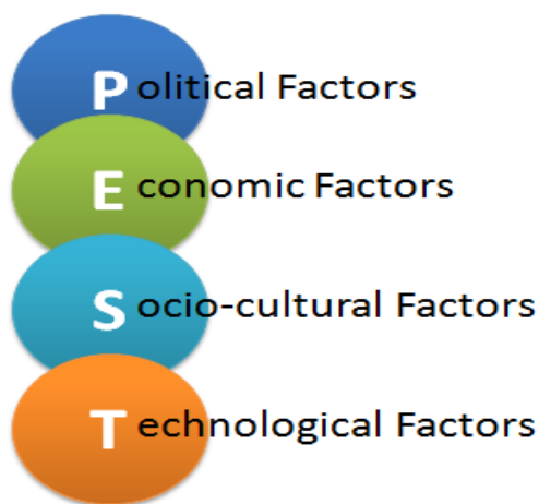
Slika 5. PEST analiza
