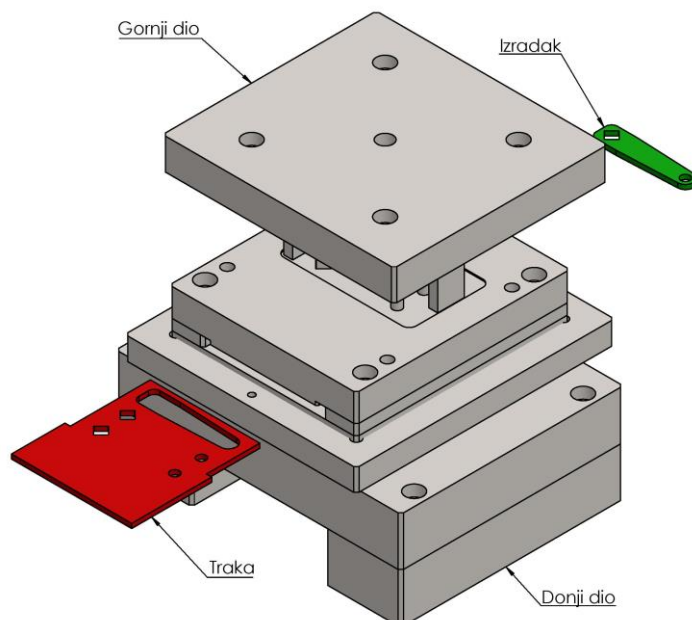
Slika 7.1 Sklop alata
