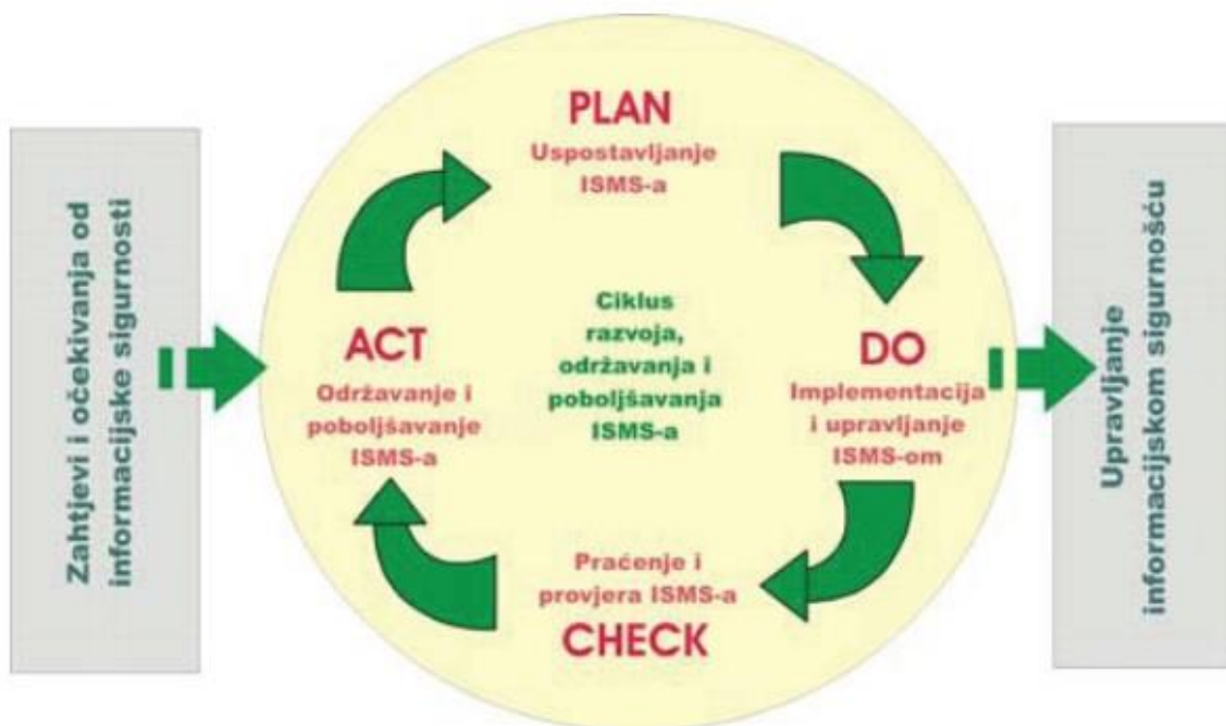
Slika 7 - PDCA ciklus
