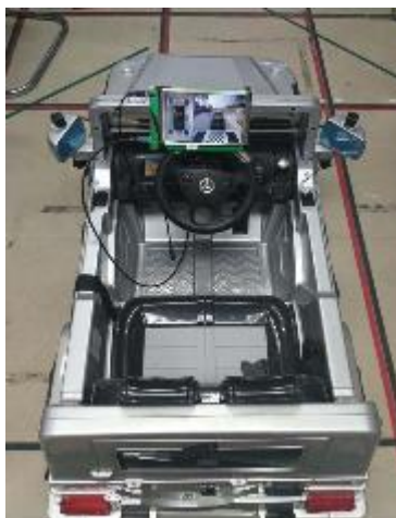
Slika 3.3 Prikaz sustava unutar vozila.
