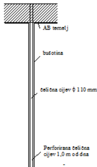
Slika 6.11. Skica temelja, bušotine i čelične cijevi
