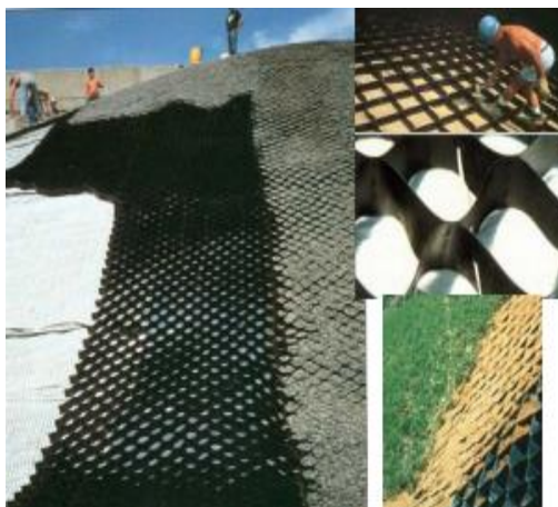
Slika2.8. Kose obaloutvrde s oblogom od sintetskih materijala ispunjenih zemljom[6]
