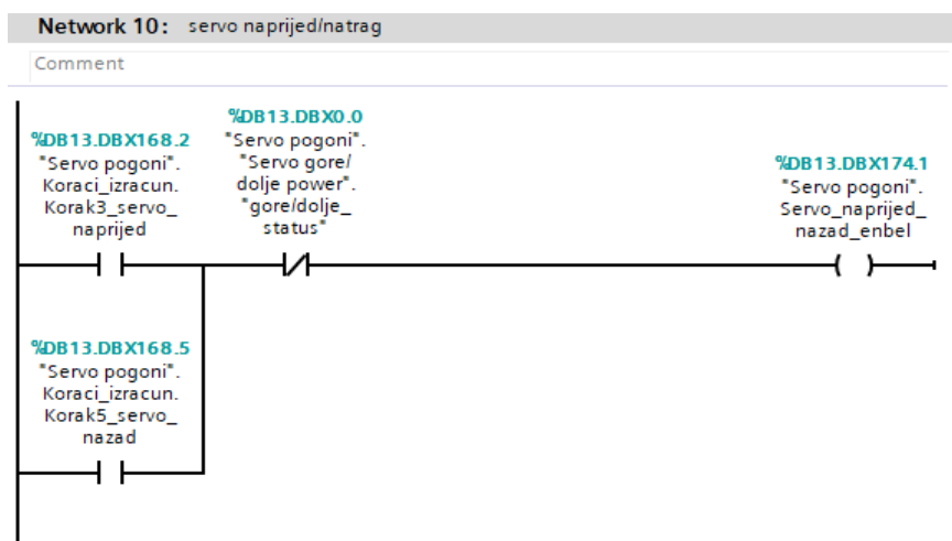
Slika 7.3.10 network 10 izlazi
