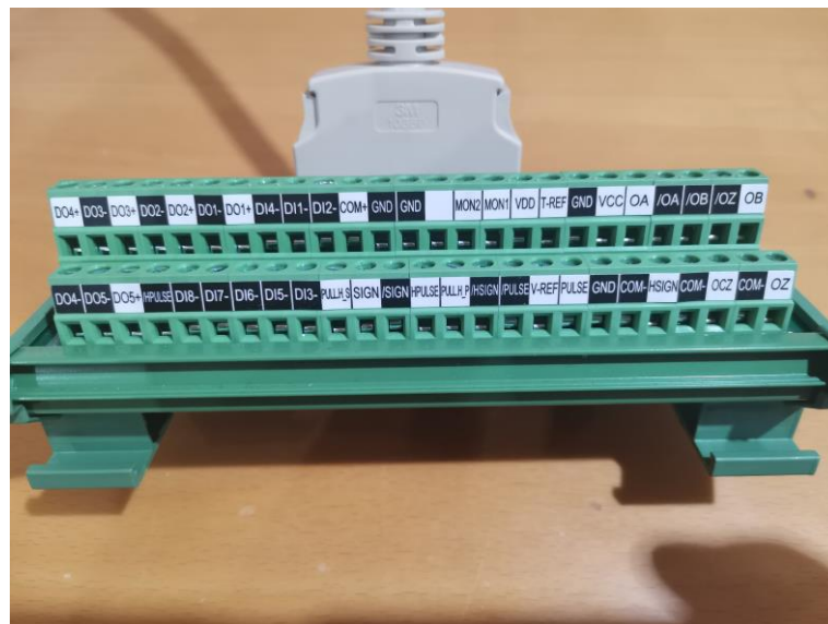
Slika 4.2 Delta pločica
