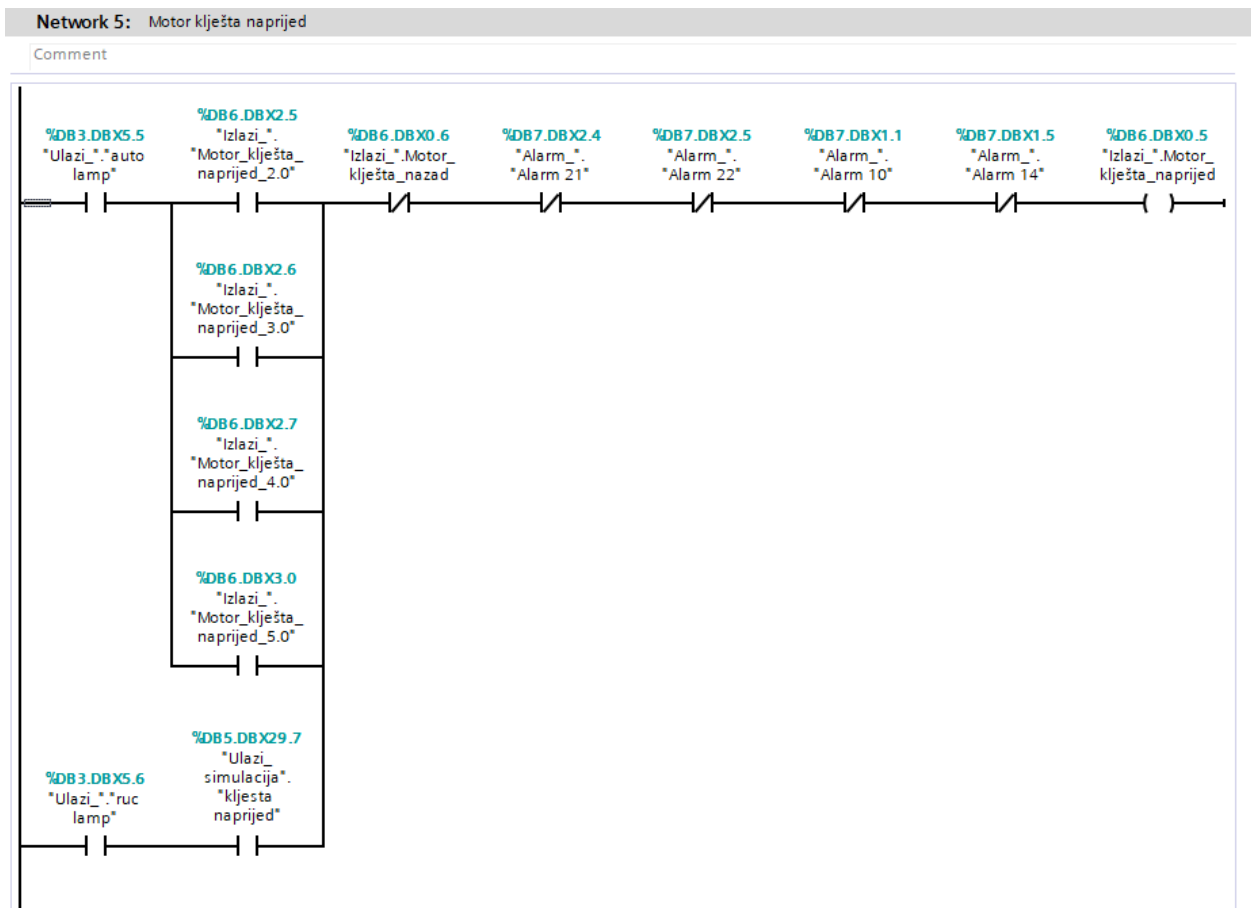
Slika 7.3.5 network 5 izlazi
