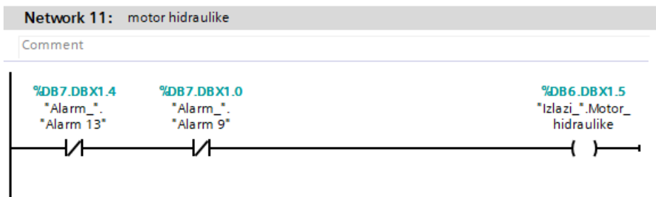
Slika 7.3.11 network 11 izlazi
