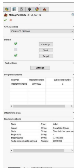
Slika 40. Izbornik za izbor postprocesora i definiranje nul-točaka
