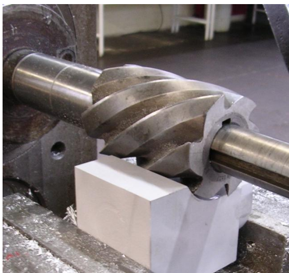
Slika 17. Protusmjerno glodanje
