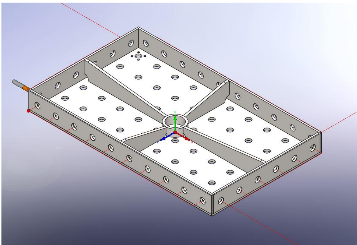
Slika 62. Simulacija glodanja bridova 0,5/45^\circ - 2. stezanje
