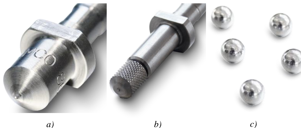
Slika 11. Indentori za standardnu Rockwell metodu, a) konični indenter, b) držač kuglica, c) karbidne kuglice [7]
