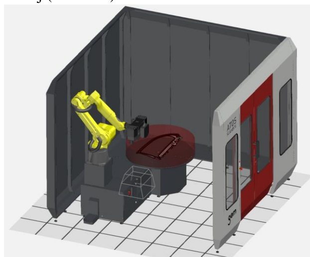
Slika 4-2 Mjerna postava
