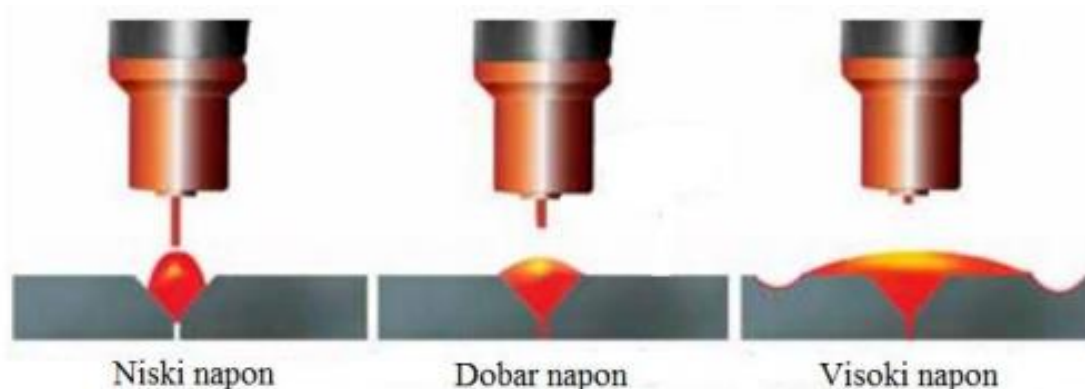
Slika 8.6 Shematski oblik zavara prema naponu električnog luka
