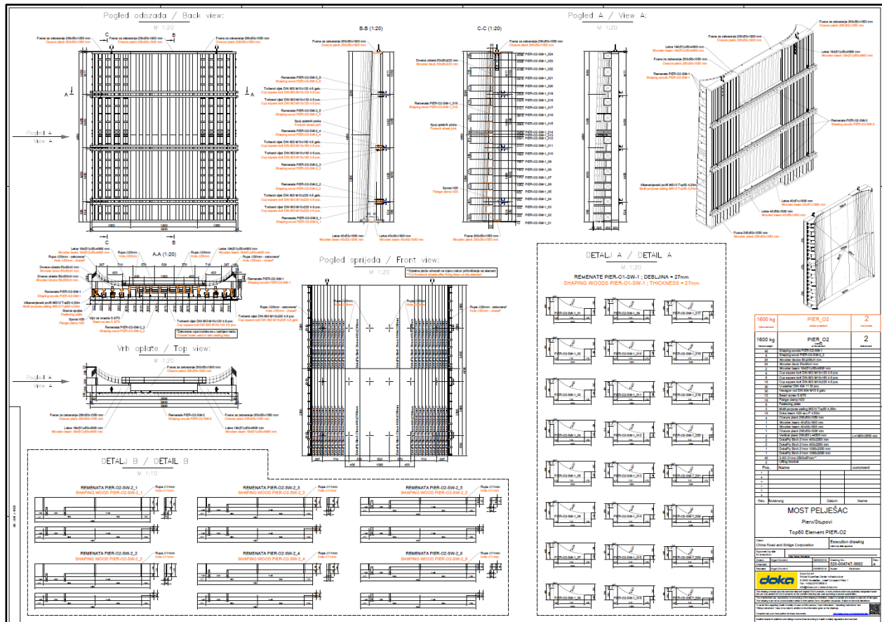
Slika 4.12. Primjer radioničkog nacrtu oplatnog elementa [8]
