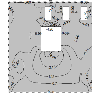
Aa - g.zona - Pravac 1 - max Aa1,g= -4.26 cm 2 /m
