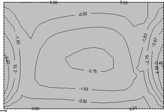
Aa - g.zona - Pravac 1 - max Aa1,g= -5.49 cm 2 /m
