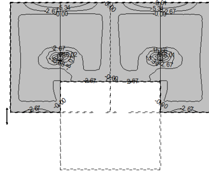
Nivo: [2.35 m] Aa - g.zona - Pramac 2 - max Aa2,g = -16.02 cm 2 /m
