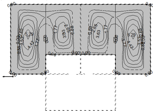
Nivo: [2.35 m] Aa - d.zona - Pravac 1 - max Aa1,d= 5.29 cm 2 /m
