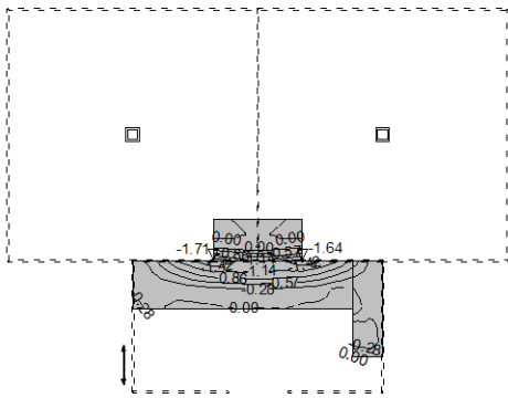
Nivo: [1.62 m] Aa - g.zona - Pravac 2 - max Aa 2,g = -1.71 cm 2 /m
