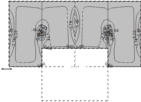
Nivo: [2.35 m] Aa - g.zona - Pramac 1 - max Aa1,g = -16.44 cm 2 /m
