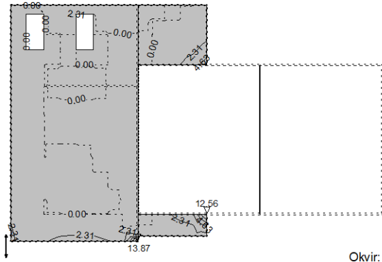
Aa - d.zona - Pravac 2 - max Aa2,d= 13.87 cm 2 /m
