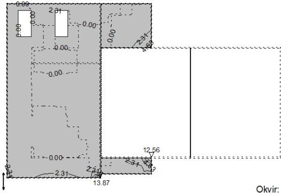
Okvir: V_2 Aa - d.zona - Pravec 2 - max Aa2,d= 13.87 cm 2 /m
