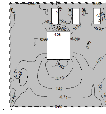
Okvir: H_3 Aa - g.zona - Pravec 1 - max Aa1,g= -4.26 cm 2 /m
