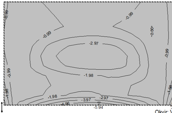
Aa - g.zona - Pravac 2 - max Aa2,g= -5.94 cm 2 /m
