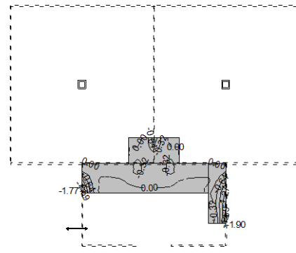
Nivo: [1.62 m] Aa - g.zona - Pravac 1 - max Aa 1,g = -1.90 cm 2 /m
