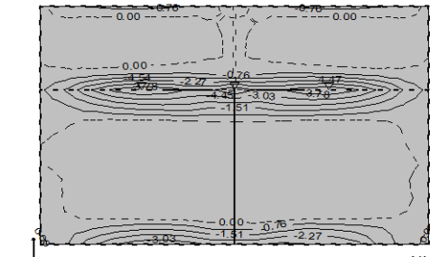
Nivo: [4.40 m] Aa - g.zona - Pravac 2 - max Aa2,g= -4.54 cm 2 /m
