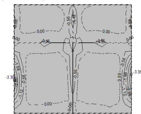
Nivo: [4.40 m] Aa - g.zona - Pravac 1 - max Aa1,g= -3.36 cm 2 /m
