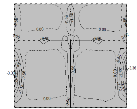
Nivo: [4.40 m] Aa - g.zona - Pramac 1 - max Aa1,g = -3.36 cm 2 /m
