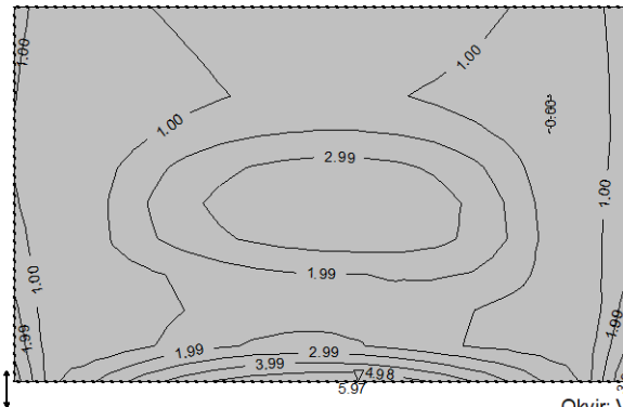
Aa - d.zona - Pravac 2 - max Aa2,d= 5.97 cm 2 /m
