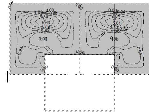
Nivo: [2.35 m] Aa - d.zona - Pramac 2 - max Aa2,d = 5.63 cm 2 /m
