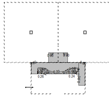
Nivo: [1.62 m] Aa - d.zona - Pravac 1 - max Aa 1,d = 0.26 cm 2 /m
