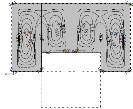
Nivo: [2.35 m] Aa - d.zona - Pramac 2 - max Aa1,d = 5.29 cm 2 /m
