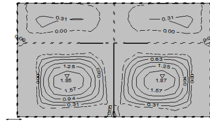
Nivo: [4.40 m] Aa - d.zona - Pramac 1 - max Aa1,d = 1.87 cm 2 /m
