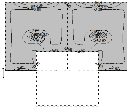
Nivo: [2.35 m] Aa - g.zona - Pravac 2 - max Aa2,g= -16.02 cm 2 /m
