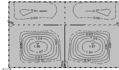
Nivo: [4.40 m] Aa - d.zona - Pravac 1 - max Aa1,d= 1.87 cm 2 /m
