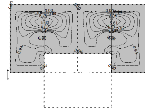
Nivo: [2.35 m] Aa - d.zona - Pravac 2 - max Aa2,d= 5.63 cm 2 /m
