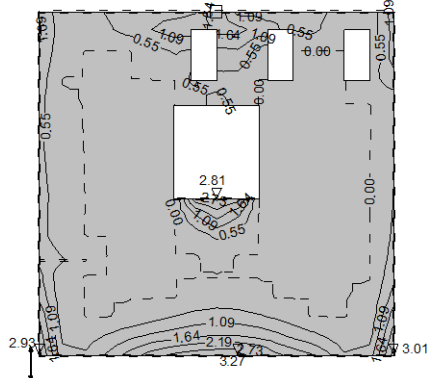
Aa - d.zona - Pravac 2 - max Aa2,d= 3.27 cm 2 /m
