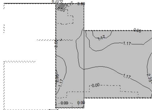
Okvir: V_5 Aa - d.zona - Pravac 1 - max Aa 1,d = 8.22 cm 2 /m
