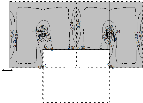
Nivo: [2.35 m] Aa - g.zona - Pravac 1 - max Aa1,g= -16.44 cm 2 /m
