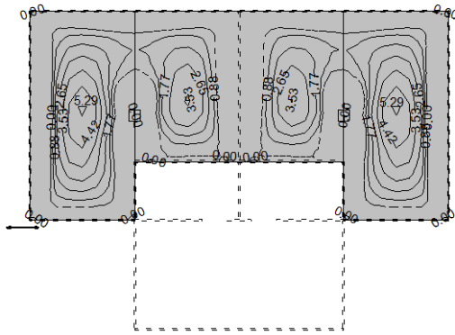
Nivo: [2.35 m] Aa - d.zona - Pramac 1 - max Aa1,d = 5.29 cm 2 /m
