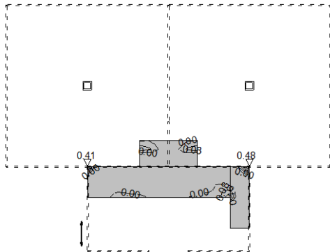
Nivo: [1.62 m] Aa - d.zona - Pravac 2 - max Aa 2,d = 0.48 cm 2 /m
