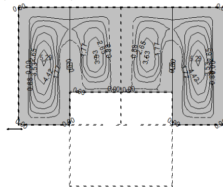
Nivo: [2.35 m] Aa - d.zona - Pravac 1 - max Aa1,d= 5.29 cm 2 /m
