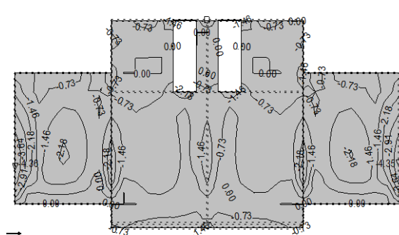
Aa - g.zona - Pravac 1 - max Aa1,g= -4.36 cm 2 /m
