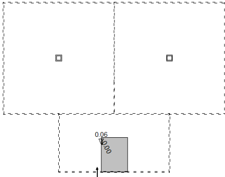
Nivo: [0.00 m] Aa - d.zona - Pravac 2 - max Aa 2,d = 0.06 cm 2 /m
