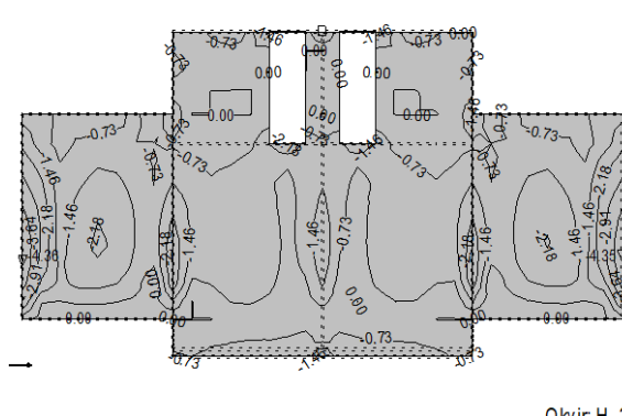
Okvir: H_2 Aa - g.zona - Pravec 1 - max Aa1,g= -4.36 cm 2 /m
