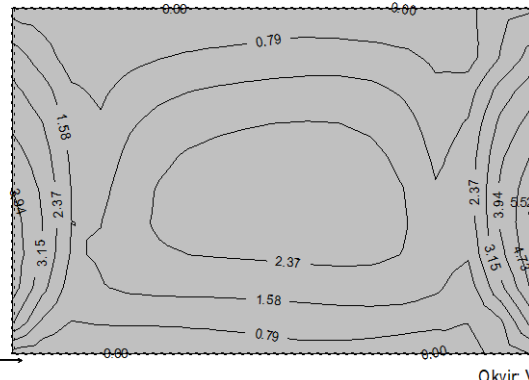
Okvir: V_4 Aa - d.zona - Pravec 1 - max Aa1,d= 5.52 cm 2 /m
