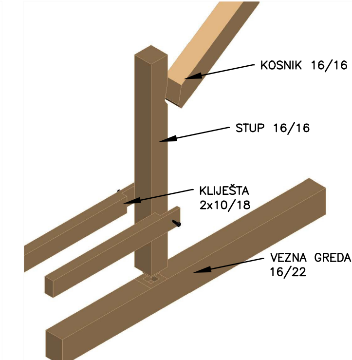
DETALJ 3 M 1:25
