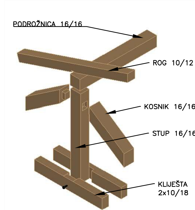
DETALJ 2 M 1:25
