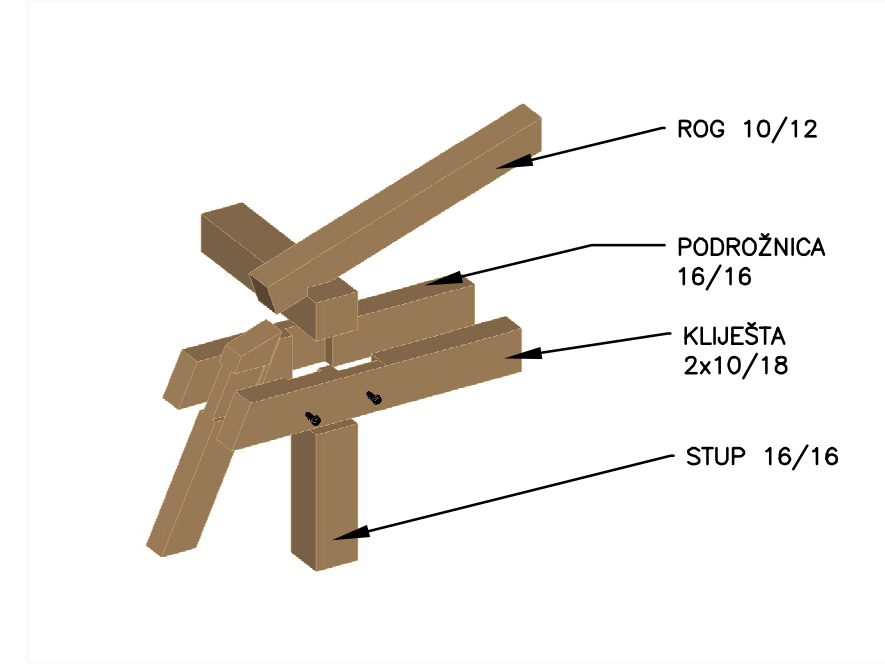
DETALJ 1 M 1:25
