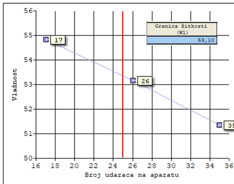
Slika 3.2. Dijagram određivanja granica plastičnost
