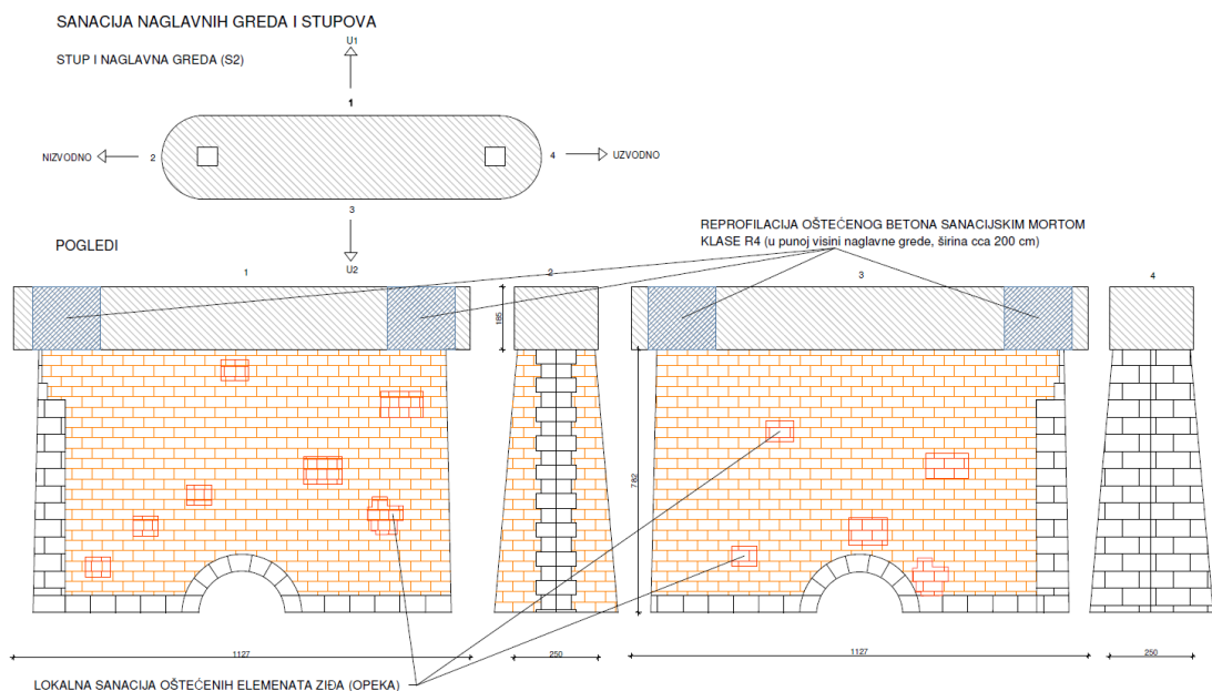
Slika 65. Nacrt sanacijskih radova naglavnih greda i stupova
