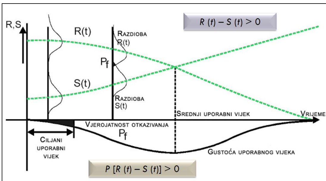
Slika 2. Probabilistička procjena uporabnog vijeka
