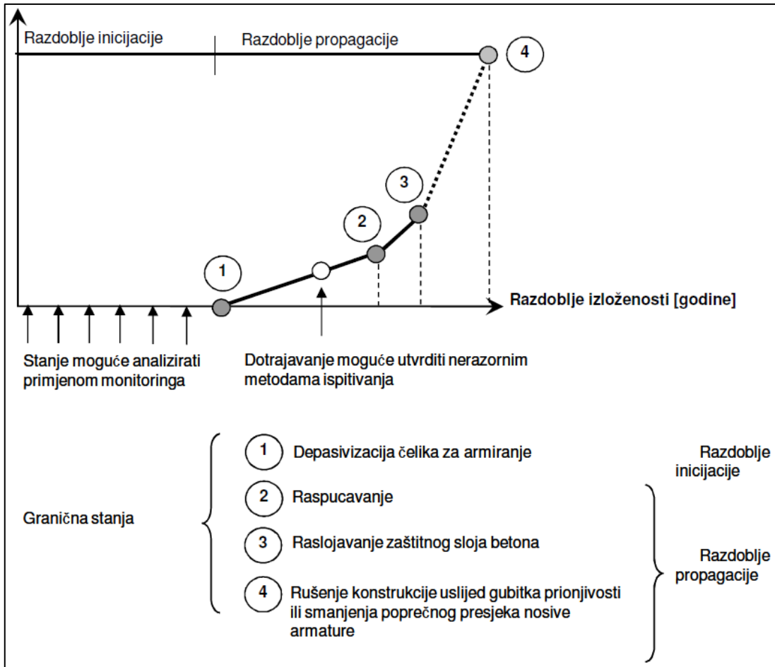
Slika 1. Trajnost konstrukcije u odnosu na gračno stanje
