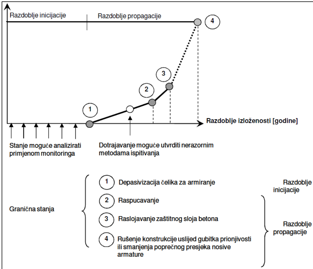
Slika 1. Trajnost konstrukcije u odnosu na granično stanje
