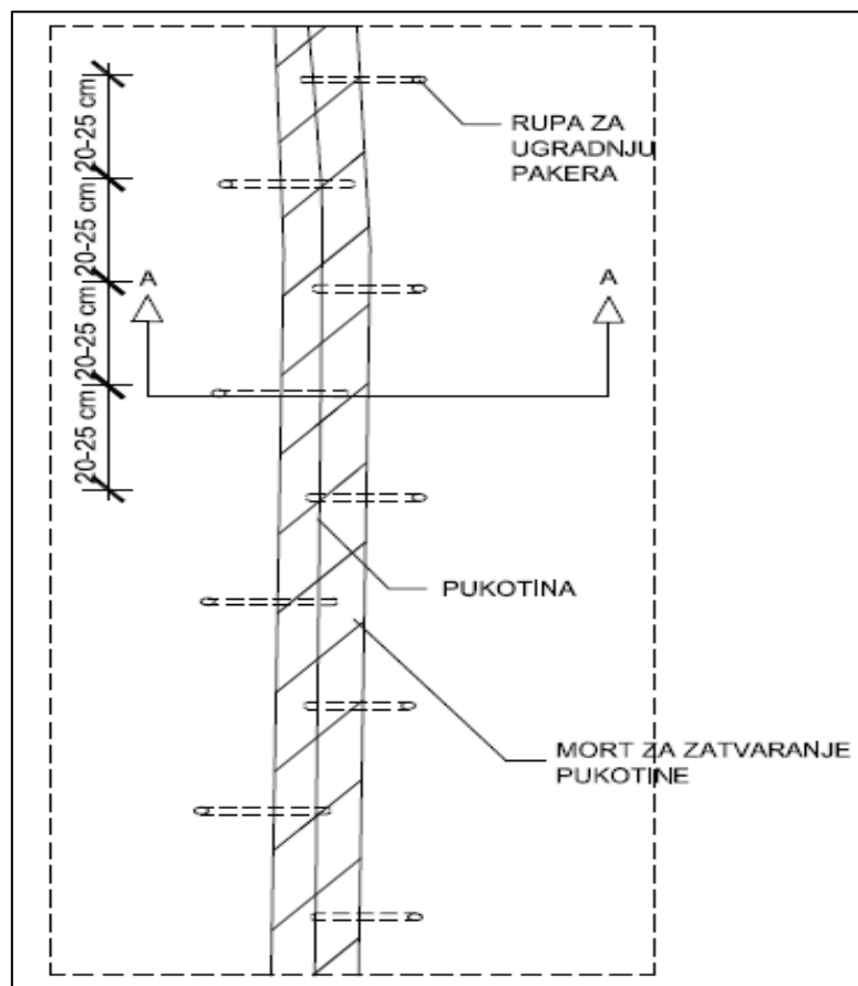
Slika 29. Detalj injektiranja bušenim pakerima pod pritiskom
