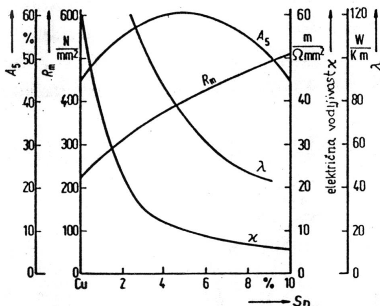
Slika 7. Dijagram mehaničkih i fizikalnih svojstva gnječenih bronca [2]
