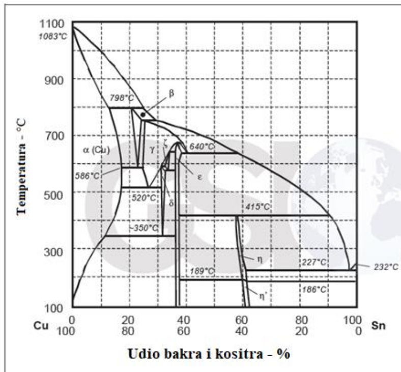
Slika 21. Dijagram ovisnosti temperature i udjela Cu i Sn [6]
