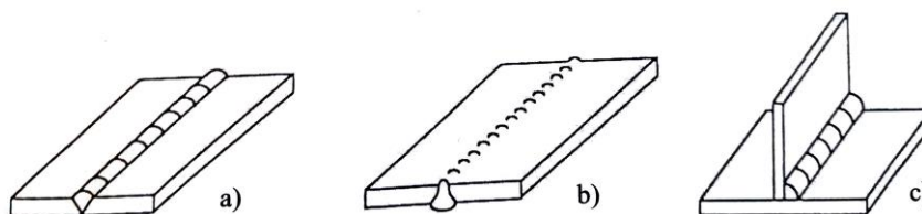
a) PA-vodoravni, b) PE-naaglavni, c) PB-vodoravno-okomiti
