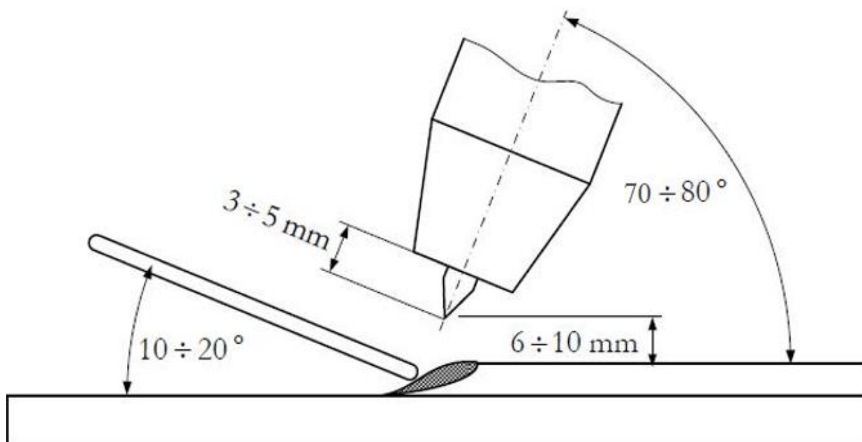
Slika 29. Položaj pištolja i dodatnog materijala u odnosu na radni komad [26, 31]
