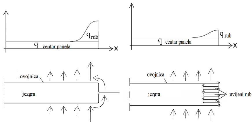
Slika 5.2.8. Shematski prikazana redukcija prolaska topline kroz rub panela
